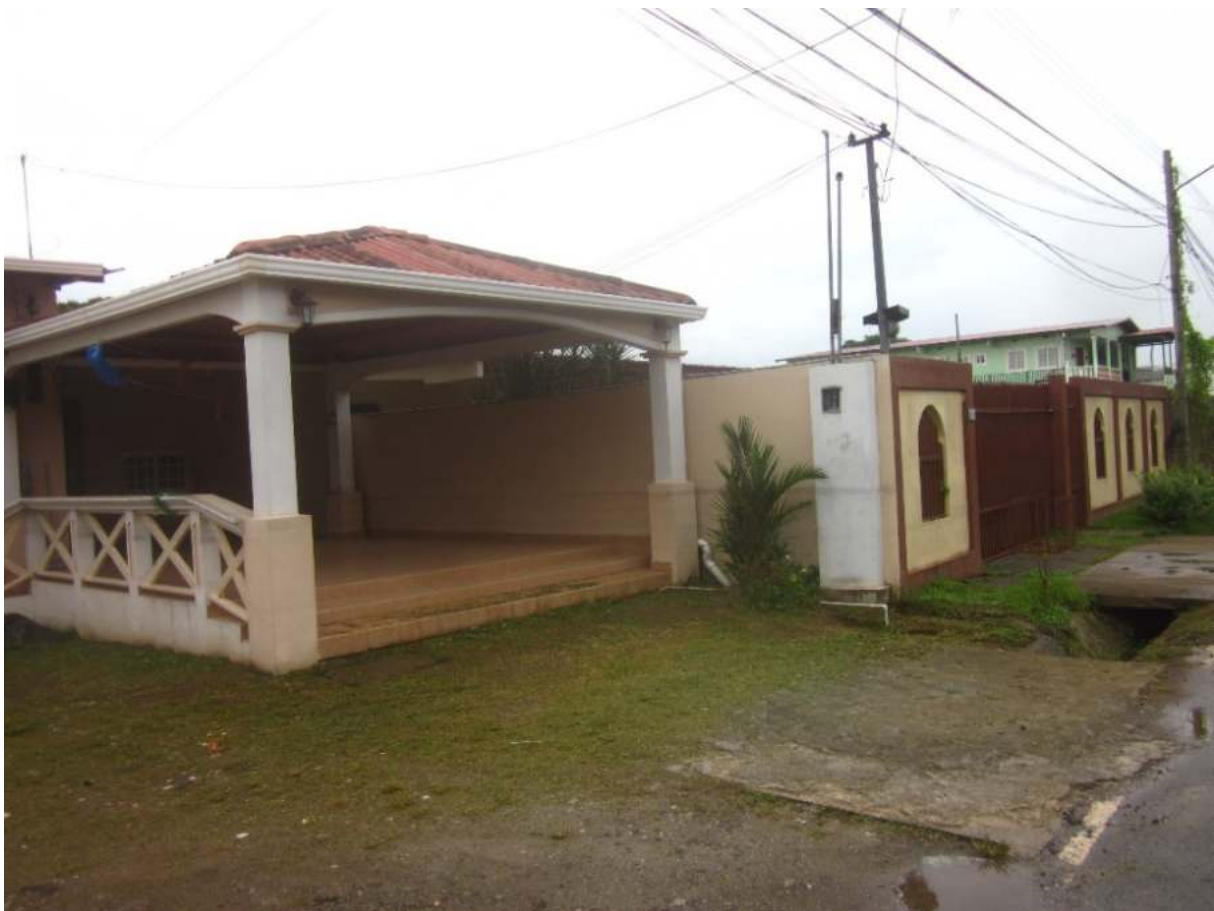
Figura 4. Ejemplo de actuación de protección (porche escalonado) frente a pequeñas inundaciones en Ciudad Radial. En la imagen se aprecia el nivel alcanzado por las aguas en las inundaciones de septiembre de 2015.
