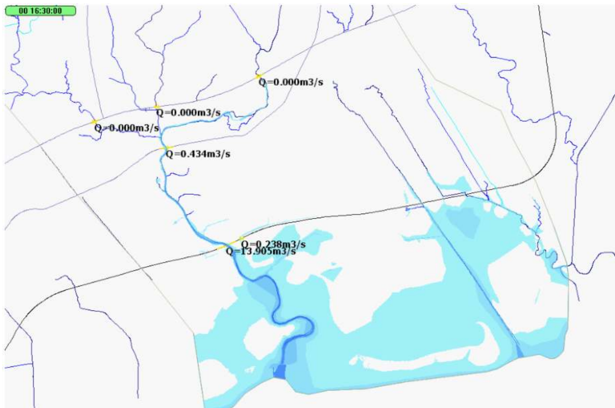
Figura 5. Inundación costera producida por una cota del nivel del mar de +3.3 m.
