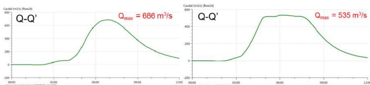
Figura 20. Hidrogramas resultantes en una sección del río en la zona de Los Pueblos con balsas de laminación libre (izquierda) y con balsas de laminación controlada (derecha).
