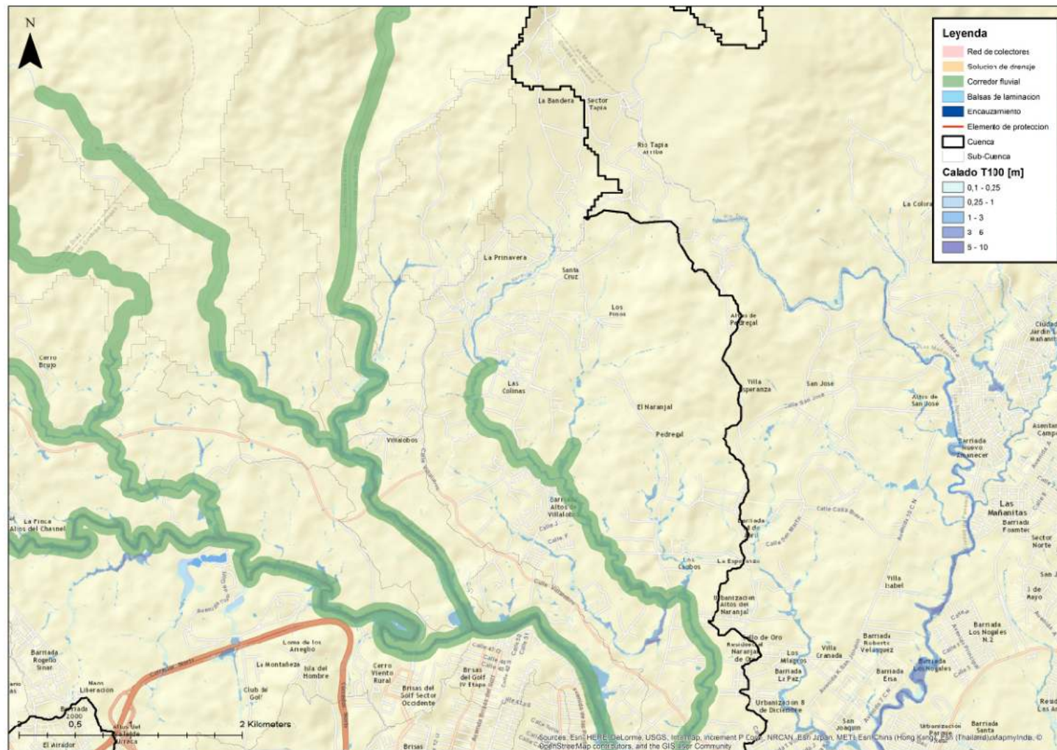
Figura 12. Plano 1-3 de actuaciones generales en la cuenca del río Juan Díaz.
